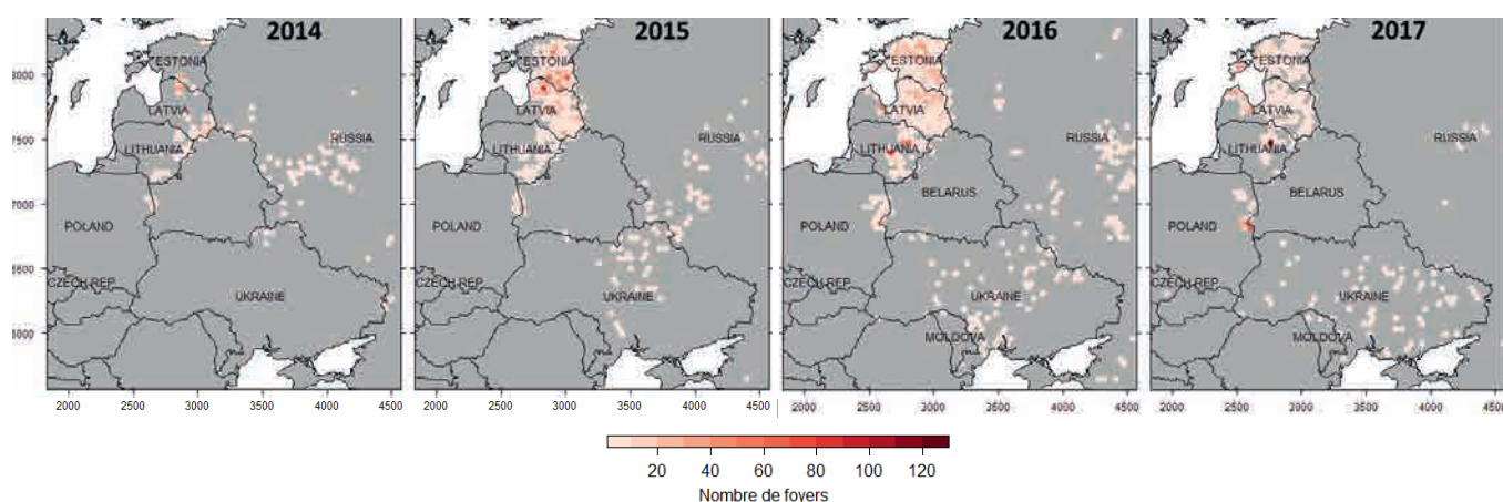
Figure 1 : Évolution des foyers et cas de Peste Porcine Africaine (PPA) chez les porcs domestiques et les sangliers sauvages dans le Nord-Est de l'Europe du 1 er janvier 2014 au 14 juin 2017 (source : ADNS/FAO Empres-i).
