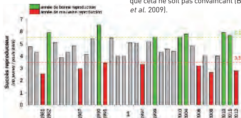
Évolution du succès reproducteur de la perdrix grise dans le centre-nord de la France de 1979 à 2012.
