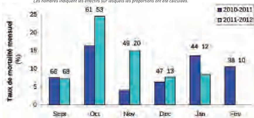
Figure 8 PROPORTION D'OISEAUX MORTS PAR MOIS.
