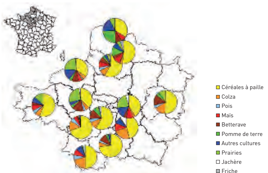
Figure 2 LOCALISATION ET ASSOLEMENT DES TREIZE SITES D'ÉTUDE.
