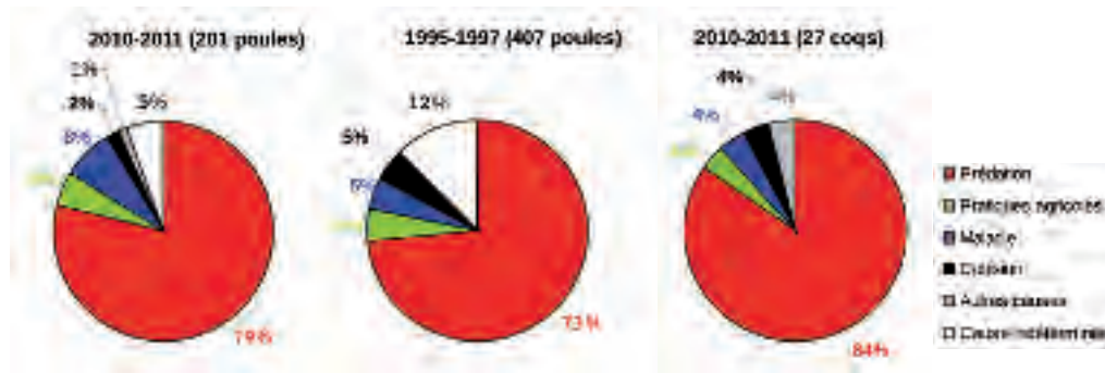
Figure 6 CAUSES DE MORTALITÉ DES PERDRIX SUIVIES PAR TÉLÉMÉTRIE AU PRINTEMPS-ÉTÉ.
