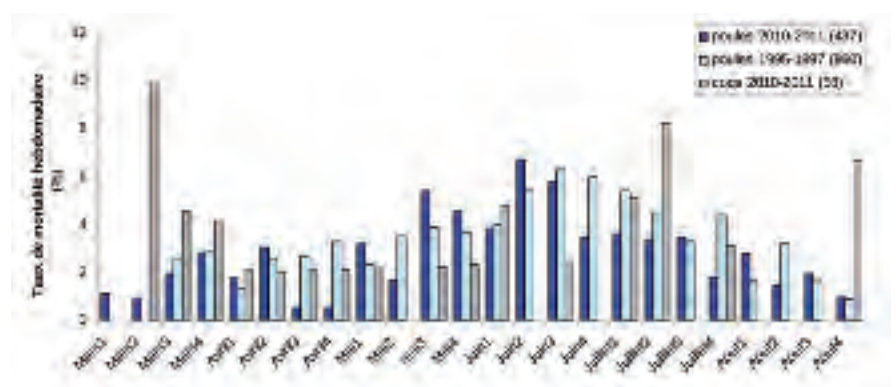
Figure 5 CHRONOLOGIE DE LA MORTALITÉ DES PERDRIX AU PRINTEMPS-ÉTÉ.
