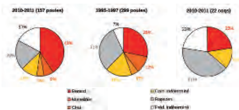
Figure 7 PRÉDATEURS IDENTIFIÉS DANS LES CAS DE PRÉDATION DE PERDRIX OBSERVÉS AU PRINTEMPS-ÉTÉ.
